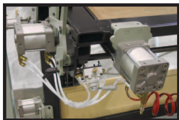
CYLINDRES PNEUMATIQUES À DOUBLE ACTION
