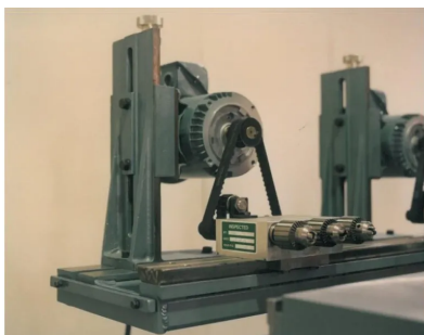
J20 - BROCHES MULTIPLES AVEC MANDRIN JACOBS
