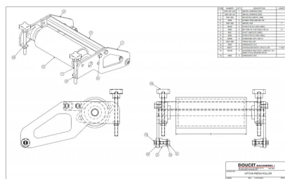
ROULEAU PRESSEUR
