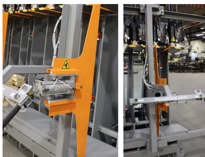
PIED PRESSEUR PNEUMATIQUE
