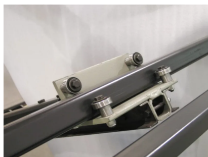
ROULEMENTS À BILLES
