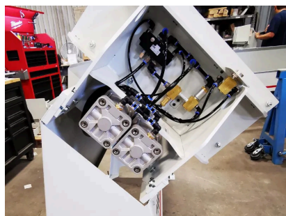
CYLINDRES PNEUMATIQUES À DOUBLE ACTION
